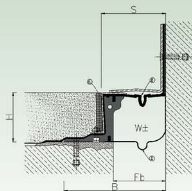
E 500/NcL-070
