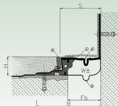
E 500/NbL
