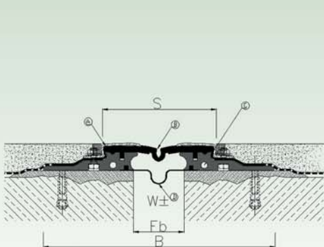
500/Na-050
