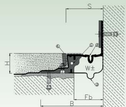
E 500/Na-050
