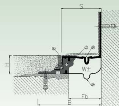
E 500/NaL-050
